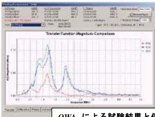
OWA による試験結果と併せて表示した、典型的な三相変圧器の伝達関数プロット
